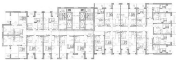
КОРПУС 1 Секция 1 План 12-16 этажей
