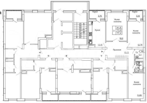
КОРПУС 3 Секция 1 План 4-21 этажей
