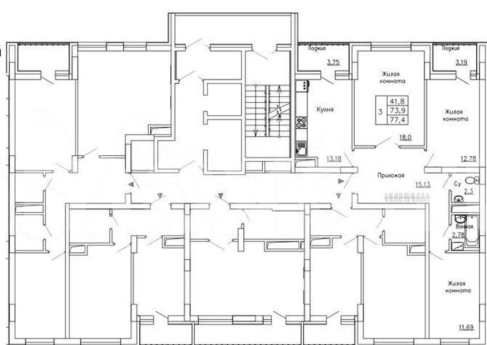
КОРПУС 3 Секция 1 План 4-21 этажей
