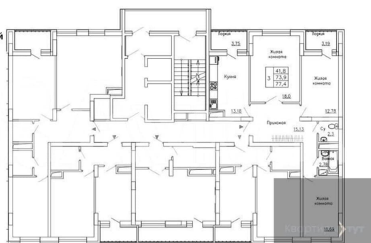
КОРПУС 3 Секция 1 План 4-21 этажей
