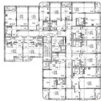
КОРПУС 1 Секция 2 План 3-8 этажей
