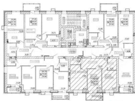
КОРПУС 5 Секция 1 План 3 этажа
