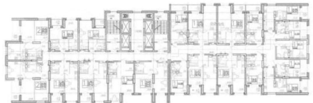
КОРПУС 1 Секция 1 План 2 этажа
