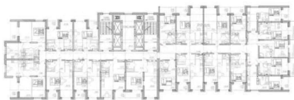
КОРПУС 1 Секция 1 План 18-19 этажей
