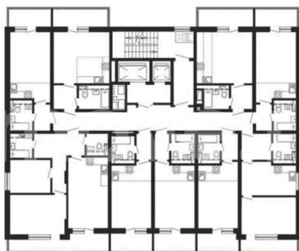
КОРПУС 1 Секция 1 План 9-16 этажей
