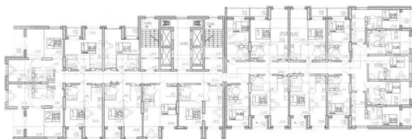
КОРПУС 1 Секция 1 План 2 этажа
