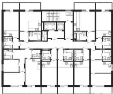
КОРПУС 1 Секция 1 План 3-8 этажей
