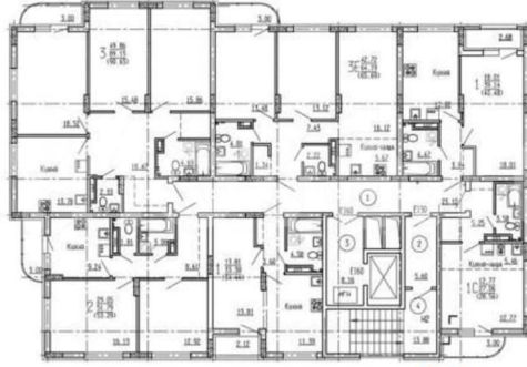
КОРПУС 2 Секция 1 План 2-9 этажей
