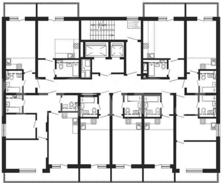
КОРПУС 1 Секция 1 План 9-16 этажей
