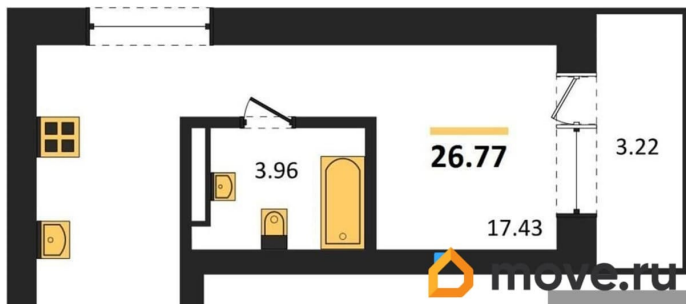
КОРПУС 1 Секция 1 План 4-11 этажей
