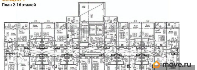
КОРПУС 6 Секция 1 План 2-16 этажей
