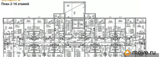
КОРПУС 6 Секция 2 План 2-16 этажей
