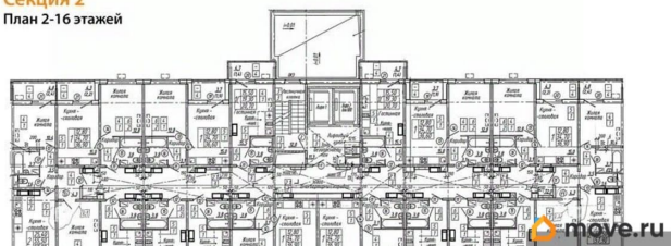
КОРПУС 6 Секция 2 План 2-16 этажей
