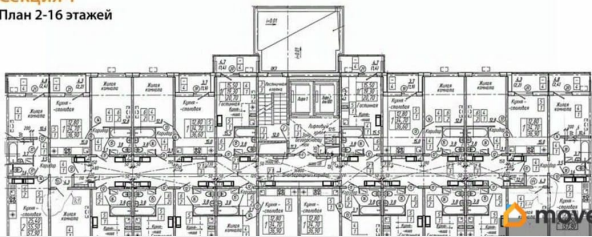
КОРПУС 6 Секция 1 План 2-16 этажей
