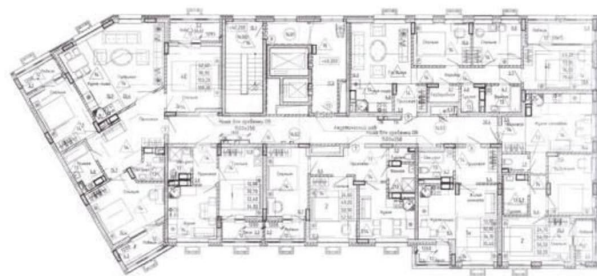
КОРПУС 3 Секция 7 План 14 этажа
