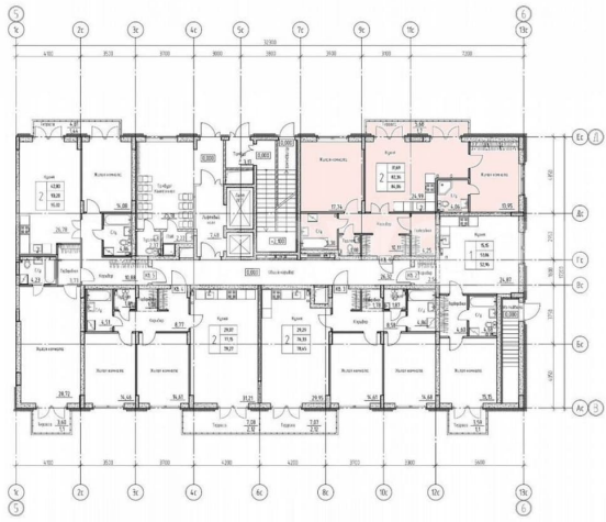
План 1 этажа
