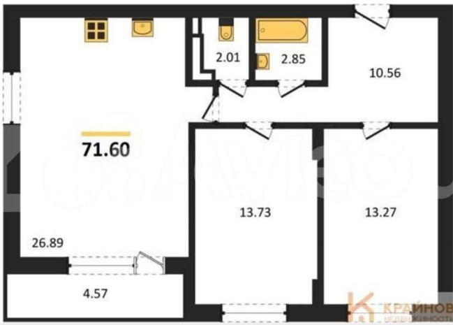
КОРПУС 2 Секция 2 План 3-17 этажей
