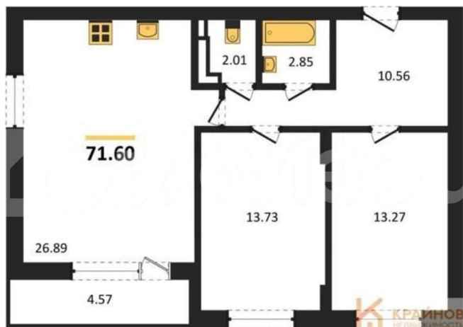
КОРПУС 2 Секция 2 План 3-17 этажей
