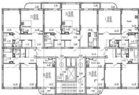
КОРПУС 2 Секция 3 План 2-9 этажей
