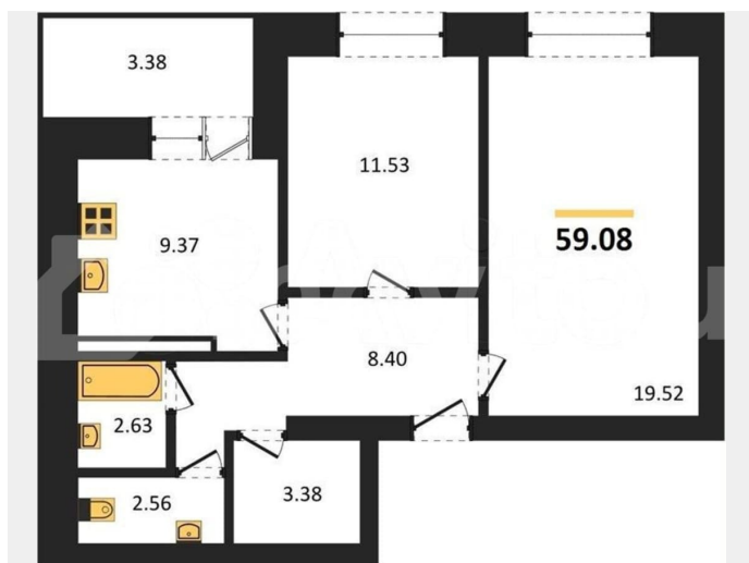
КОРПУС 2 Секция 1 План 2-10 этажей
