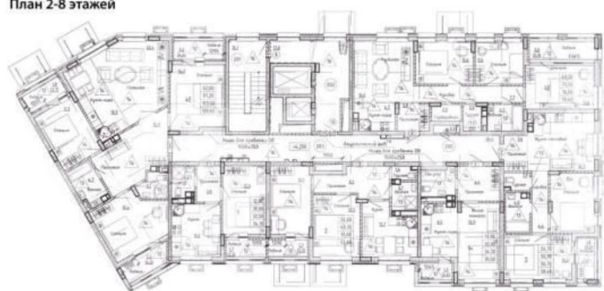
КОРПУС 3 Секция 7 План 2-8 этажей
