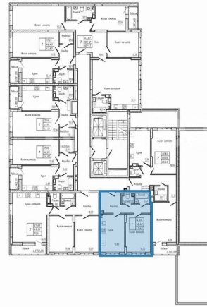
План этажа
